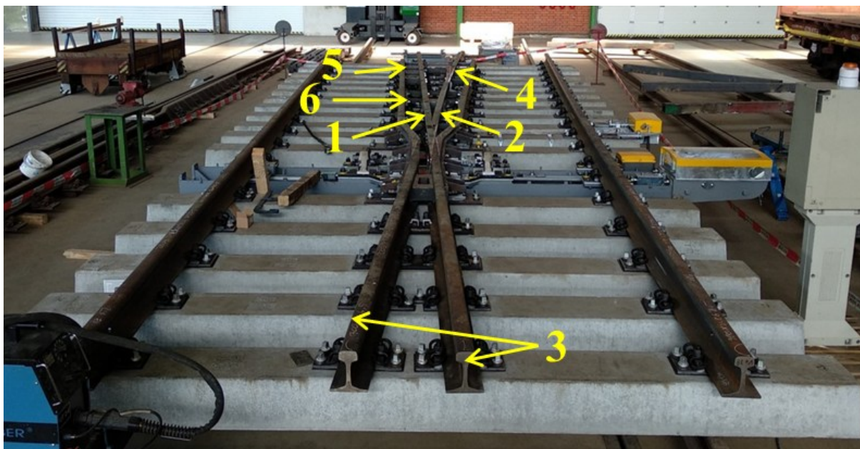
Obrázek 1 – Srdcovka s PHS s rámem z kolejnic
